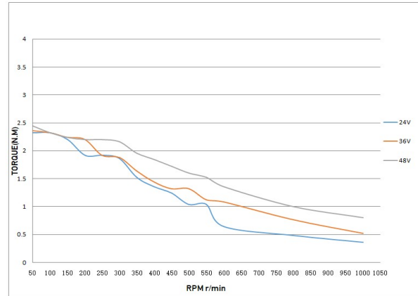
ISS57R350EA
