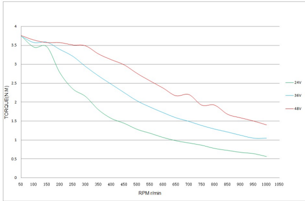
ISS86R250BR00
