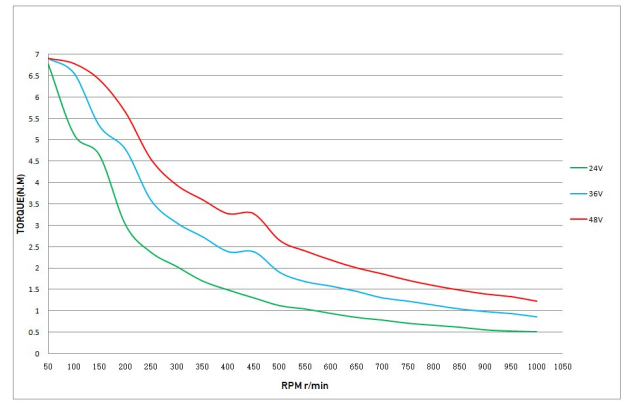
ISS86R250DR00
